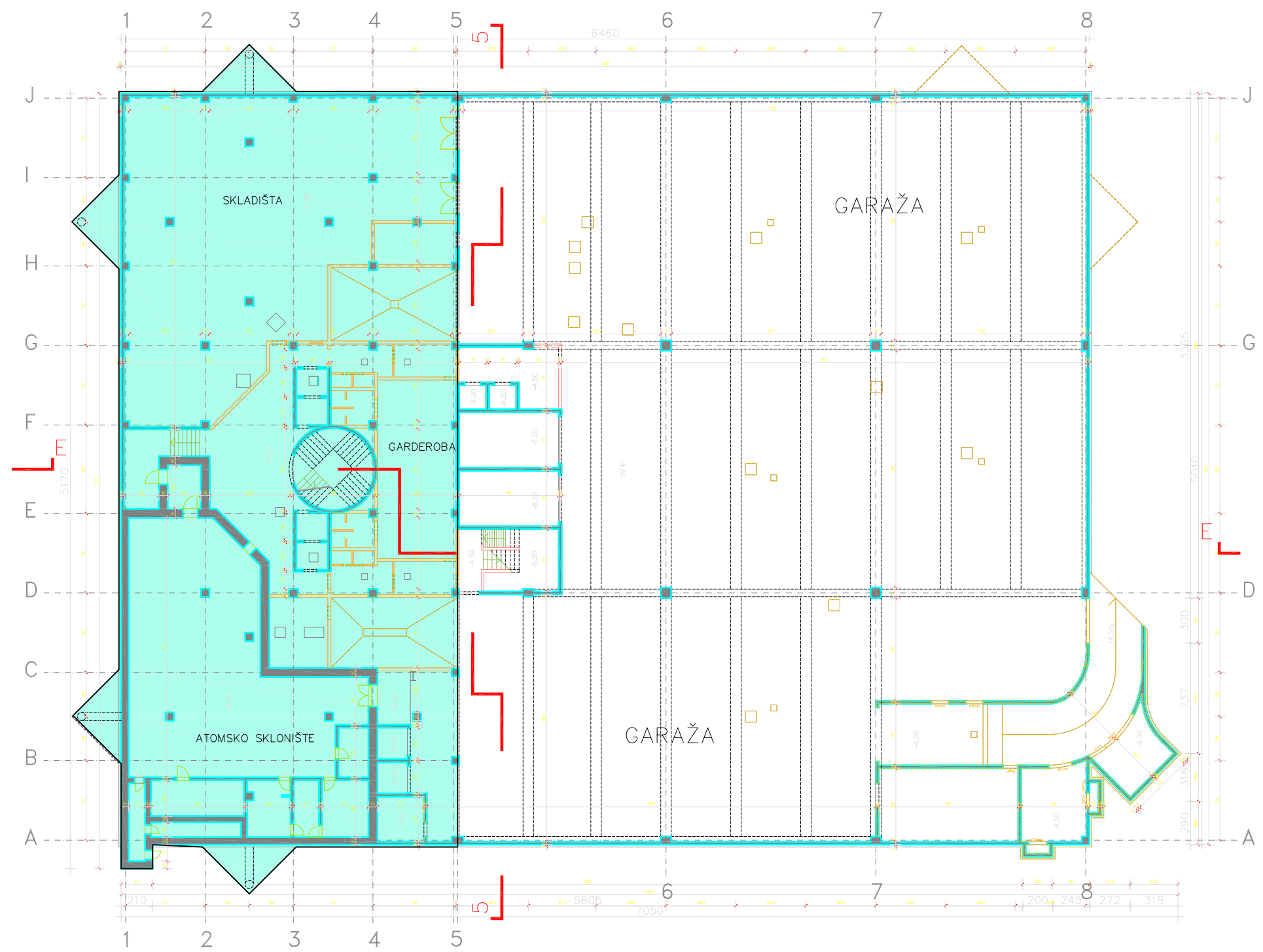
TLOCRT KARAKTERISTIČNE ETAŽE GARAŽA
